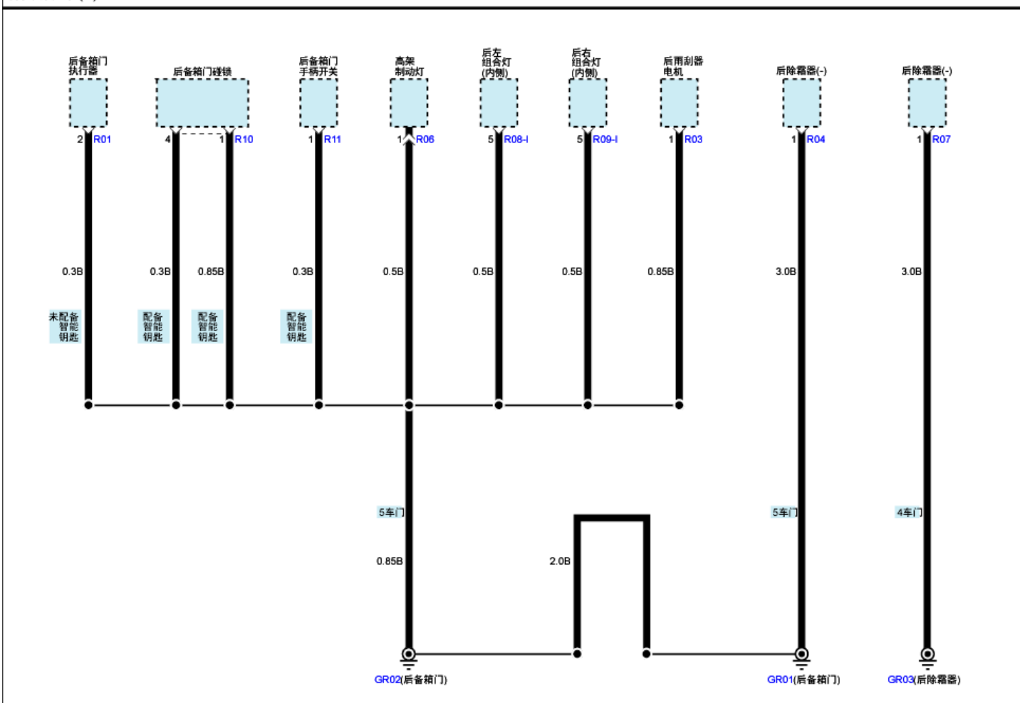
搭铁分布(6)
